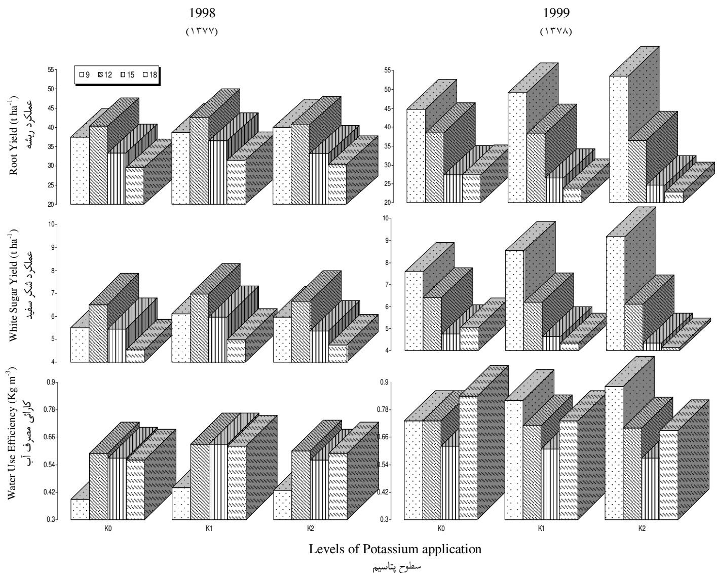
شکل ۱ تغییرات عملکرد ریشه، عملکرد شکر سفید و کارائی مصرف آب برای تولید شکر سفید در دوره‌های مختلف آبیاری (۹، ۱۲، ۱۵ و ۱۸ روز) و سطوح پتاسیم ( K_0 = عدم مصرف پتاسیم، K_1 = مصرف پتاسیم جهت رساندن پتاسیم خاک تا پنج درصد CEC خاک و K_2 = مصرف پتاسیم به میزان K_1 به اضافه نیاز گیاه) در سال‌های ۱۳۷۷ و ۱۳۷۸ - طرق
