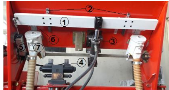
شکل ۱ مکانیسم عملگر هیدرولیکی محرک دریاچه موزعها در دستگاه فاروئر-کودکار چهار ردیفه با سامانه کنترلی ابداعی، شامل: ۱- صفحه محرک دریاچهها ۲- ریلهای حرکت صفحه ۳- جک (عملگر) هیدرولیکی دوطرفه ۴- شیر هیدرولیک برقی ۵- حسگر موقعیت دریاچه ۶- دریاچه موزع ۷- موزع کود
