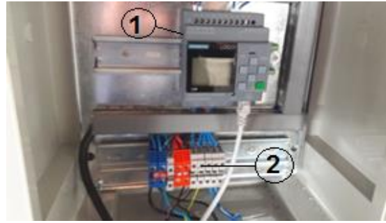
شکل ۴ محفظه (جعبه) اجزاء واحد کنترل الکترونیکی در دستگاه فاروئر-کودکار چهار ردیفه با سامانه کنترلی ابداعی، شامل ۱-PLC ۲- اتصالات (کانکتورها)
