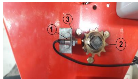
شکل ۲ محل قرارگیری حسگر موقعیت دریاچه و اجزا آن در دستگاه فاروئر-کودکار چهار ردیفه با سامانه کنترلی ابداعی، شامل: ۱- موزع ۲- حسگر ۳- دریاچه موزع
